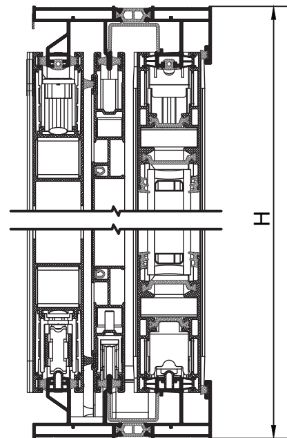
II → Χωνευτό Φιλητό Συρόμενο με 45° κοπή με Σήτα και Παντζούρι Meeting Stile Pocket Sliding 45° Cut with Flyscreen and Shutter
