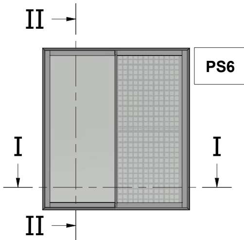
Two Sash Parallel Sliding Window 90 Degrees Cut with Narrow Interlock and Flyscreen Δίφυλλο Επάλληλο Συρόμενο με κοπή 90 μοιρών, Στενό Γάντζο και Σήτα
