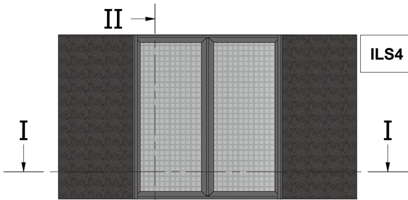
II → Χωνευτό Φιλητό Συρόμενο με 45° κοπή με Σήτα και Παντζούρι Meeting Stile Pocket Sliding 45° Cut with Flyscreen and Shutter
