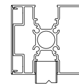
/ Κολόνα 80x80mm, απλή ή γωνιακή, συνδυαζόμενη με τάπες ή κουπαστή αλουμινίου, ειδικού σχεδιασμού και με κρυφά σημεία σύνδεσης. (03)
