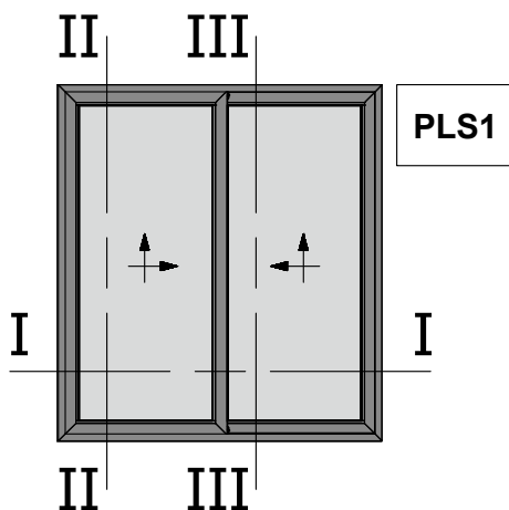
Two Sash Parallel Lift and Slide 45 Degrees Cut Right Opening Window Δίφυλλο Επάλληλο Δεξιά Ανάσυρόμενο με κοπή 45 μοιρών
