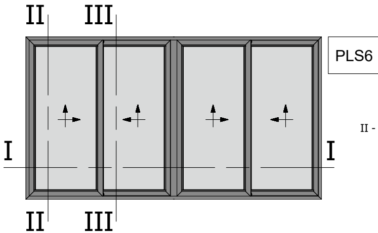
Four Sash Parallel Lift and Slide 45 Degrees Cut Right Opening Window Τετράφυλλο Επάλληλο Δεξιά Ανάσυρόμενο με κοπή 45 μοιρών
