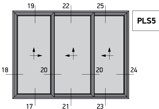
Three Sash Parallel Lift and Slide 45° Cut Right Opening Window Τρίφυλλο Επάλληλο Δεξιά Ανάσπόμενο με κοπή 45°
