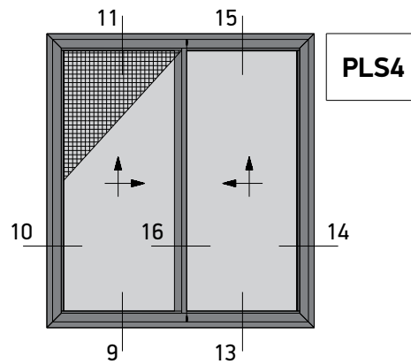
Two Sash Parallel Lift and Slide 90° Cut Right Opening Window with Flyscreen Δίφυλλο Επάλληλο Δεξιά Ανάσπόμενο με κοπή 90° με Σήτα
