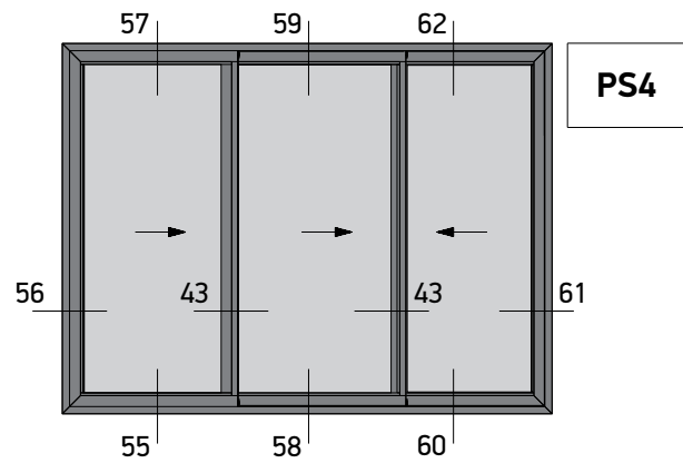
Three Sash Sliding 90° Cut Right Opening Window Τρίφυλλο Επάλληλο Δεξιά Συρόμενο με κοπή 90°
