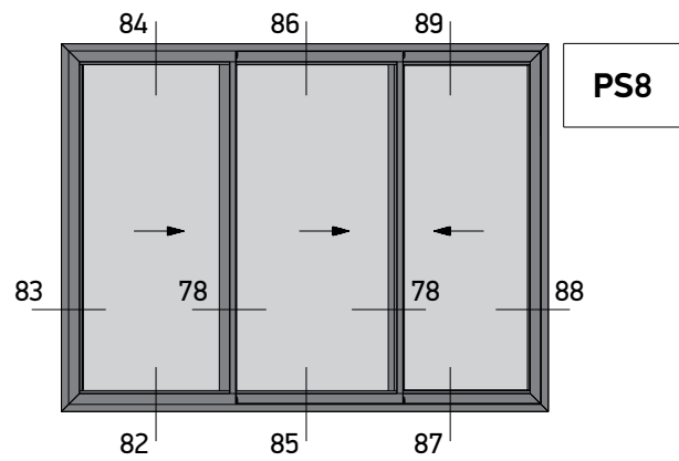
Three Sash Sliding 90° Cut Right Opening Window with Sash M4544 Τρίφυλλο Επάλληλο Δεξιά Συρόμενο με κοπή 90° με φύλλο M4544
