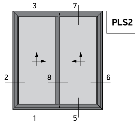
Two Sash Parallel Lift and Slide 90° Cut Right Opening Window Δίφυλλο Επάλληλο Δεξιά Ανάσπόμενο με κοπή 90°
