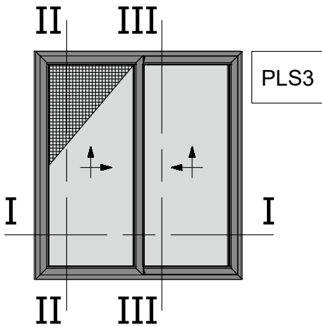
Two Sash Parallel Lift and Slide 45 Degrees Cut Right Opening Window with Flyscreen Δίφυλλο Επάλληλο Δεξιά Ανάσυρόμενο με κοπή 45 μοιρών και Σήτα
