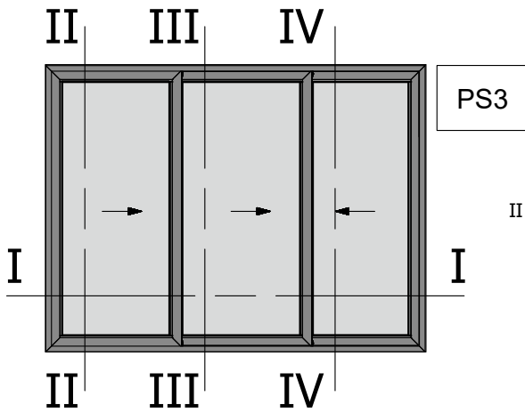
Three Sash Sliding 45 Degrees Cut Right Opening Window Τρίφυλλο Επάλληλο Δεξιά Συρόμενο με κοπή 45 μοιρών
