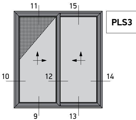
Two Sash Parallel Lift and Slide 45° Cut Right Opening Window with Flyscreen Δίφυλλο Επάλληλο Δεξιά Ανάσπόμενο με κοπή 45° και Σήτα
