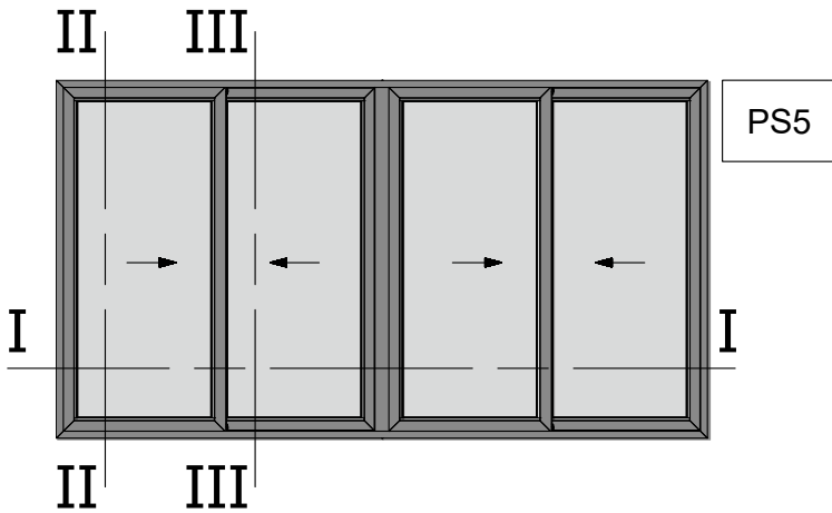
Four Sash Parallel Sliding 45 Degrees Cut Right Opening Window Τετράφυλλο Επάλληλο Δεξιά Συρόμενο με κοπή 45 μοιρών
