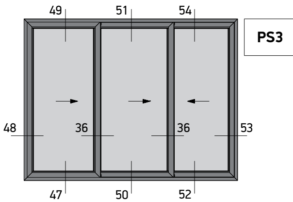
Three Sash Sliding 45° Cut Right Opening Window Τρίφυλλο Επάλληλο Δεξιά Συρόμενο με κοπή 45°
