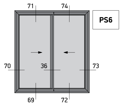
Two Sash Parallel Sliding 45° Cut Right Opening Window with sash M4542 Δίφυλλο Επάλληλο Δεξιά Συρόμενο με κοπή 45° με φύλλο M4542
