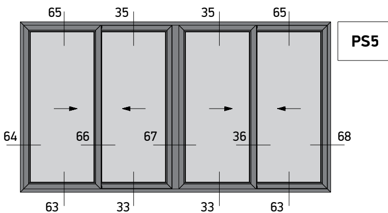
Four Sash Parallel Sliding 45° Cut Right Opening Window Τετράφυλλο Επάλληλο Δεξιά Συρόμενο με κοπή 45°
