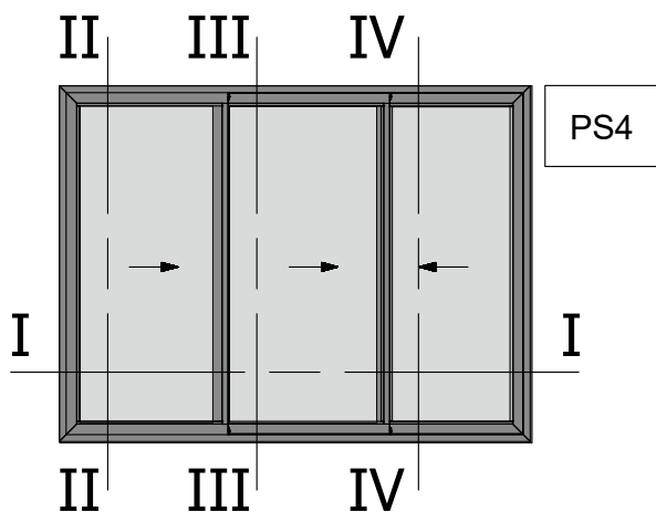
Three Sash Sliding 90 Degrees Cut Right Opening Window Τρίφυλλο Επάλληλο Δεξιά Συρόμενο με κοπή 90 μοιρών
