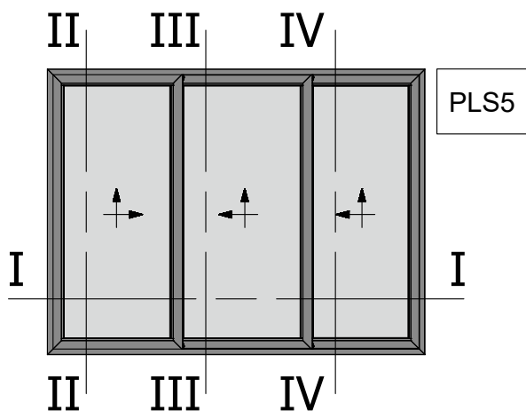
Three Sash Parallel Lift and Slide 45 Degrees Cut Right Opening Window Τρίφυλλο Επάλληλο Δεξιά Ανάσυρόμενο με κοπή 45 μοιρών
