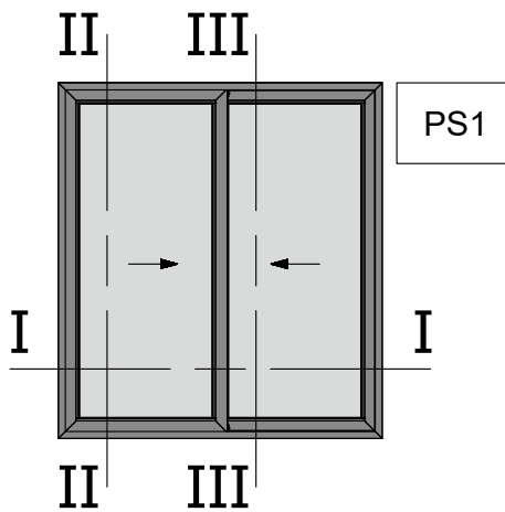
Two Sash Parallel Sliding 45 Degrees Cut Right Opening Window Δίφυλλο Επάλληλο Δεξιά Συρόμενο με κοπή 45 μοιρών
