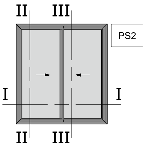
Two Sash Parallel Sliding 90 Degrees Cut Right Opening Window Δίφυλλο Επάλληλο Δεξιά Συρόμενο με κοπή 90 μοιρών
