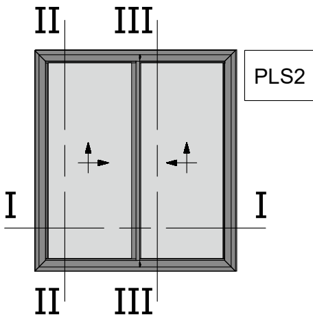
Two Sash Parallel Lift and Slide 90 Degrees Cut Right Opening Window Δίφυλλο Επάλληλο Δεξιά Ανάσυρόμενο με κοπή 90 μοιρών
