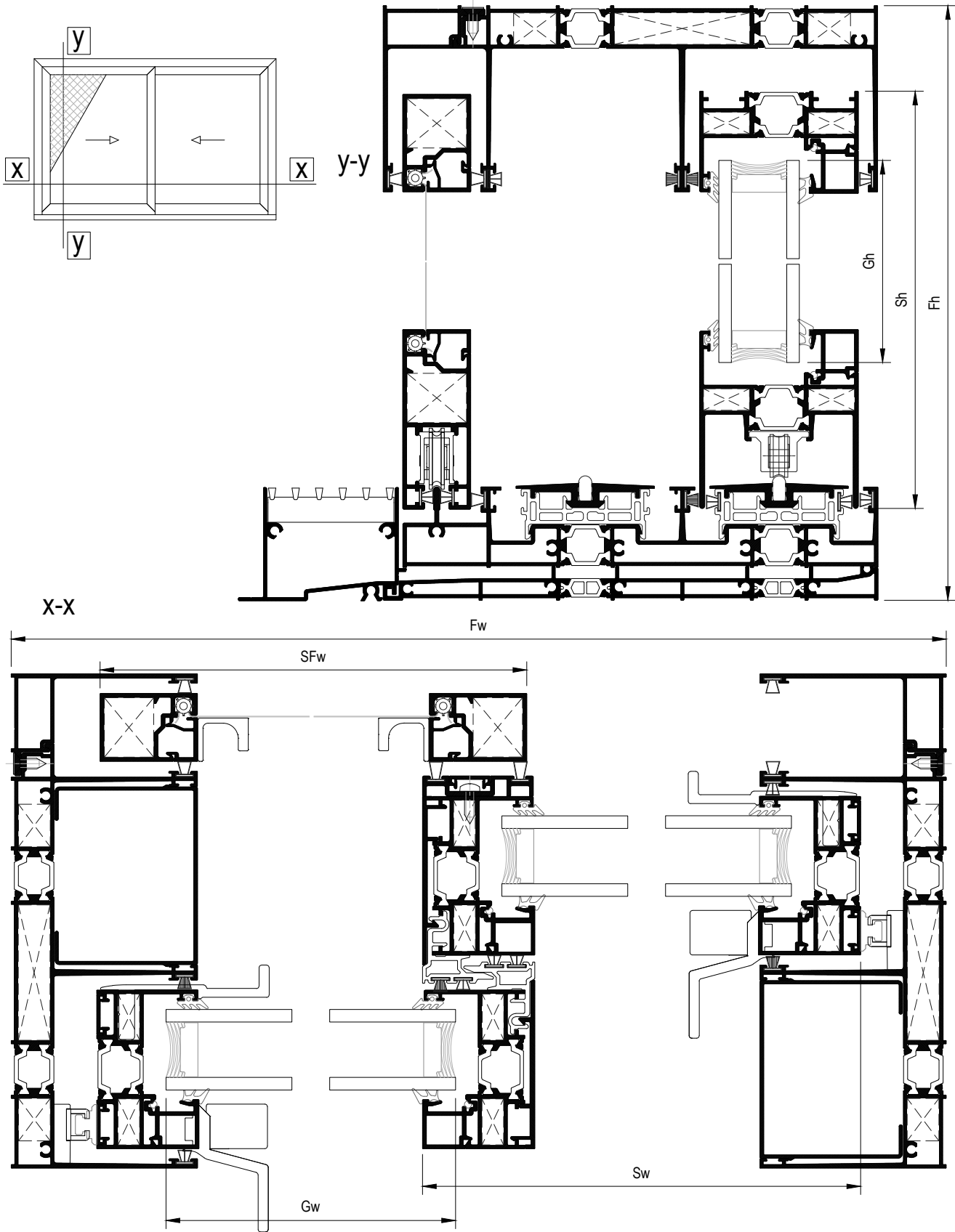
Afg Two-sash sliding window with flyscreen and gutter Δίφυλλο επάλληλο συρόμενο με σήτα και υδατολεκάνη
