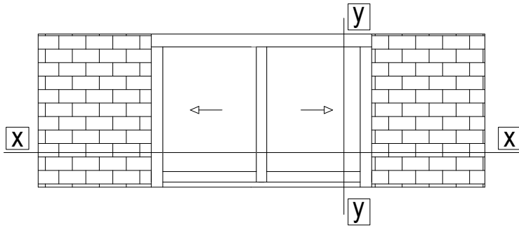
K Δίφυλλο φιλητό χωνευτό Two sash with meeting stile pocket window
