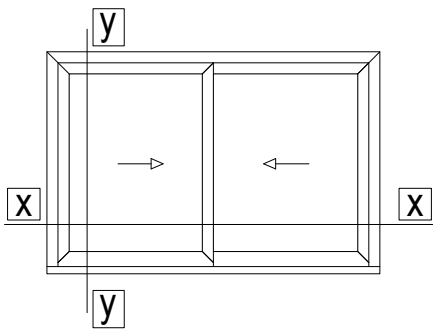
Ag Two-sash sliding window with gutter Δίφυλλο επάλληλο συρόμενο με υδατολεκάνη
