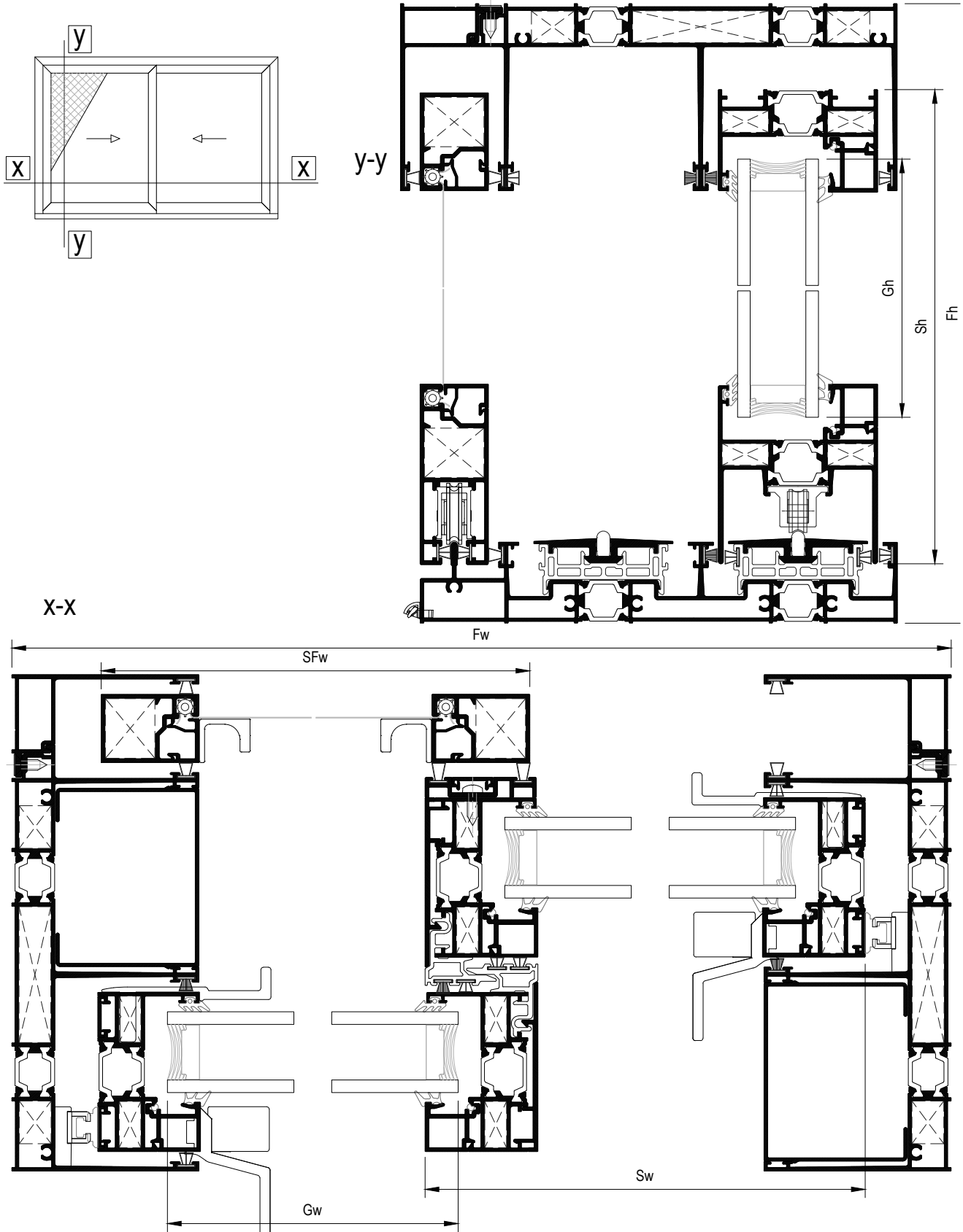
Af Two-sash sliding window with flyscreen Δίφυλλο επάλληλο συρόμενο με σήτα
