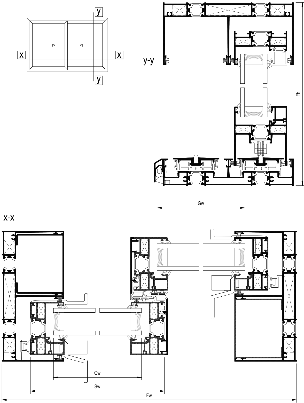
A Two-sash sliding window Δίφυλλο επάλληλο συρόμενο
