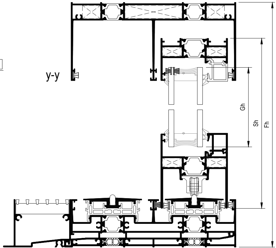
Ag Two-sash sliding window with gutter Δίφυλλο επάλληλο συρόμενο με υδατολεκάνη
