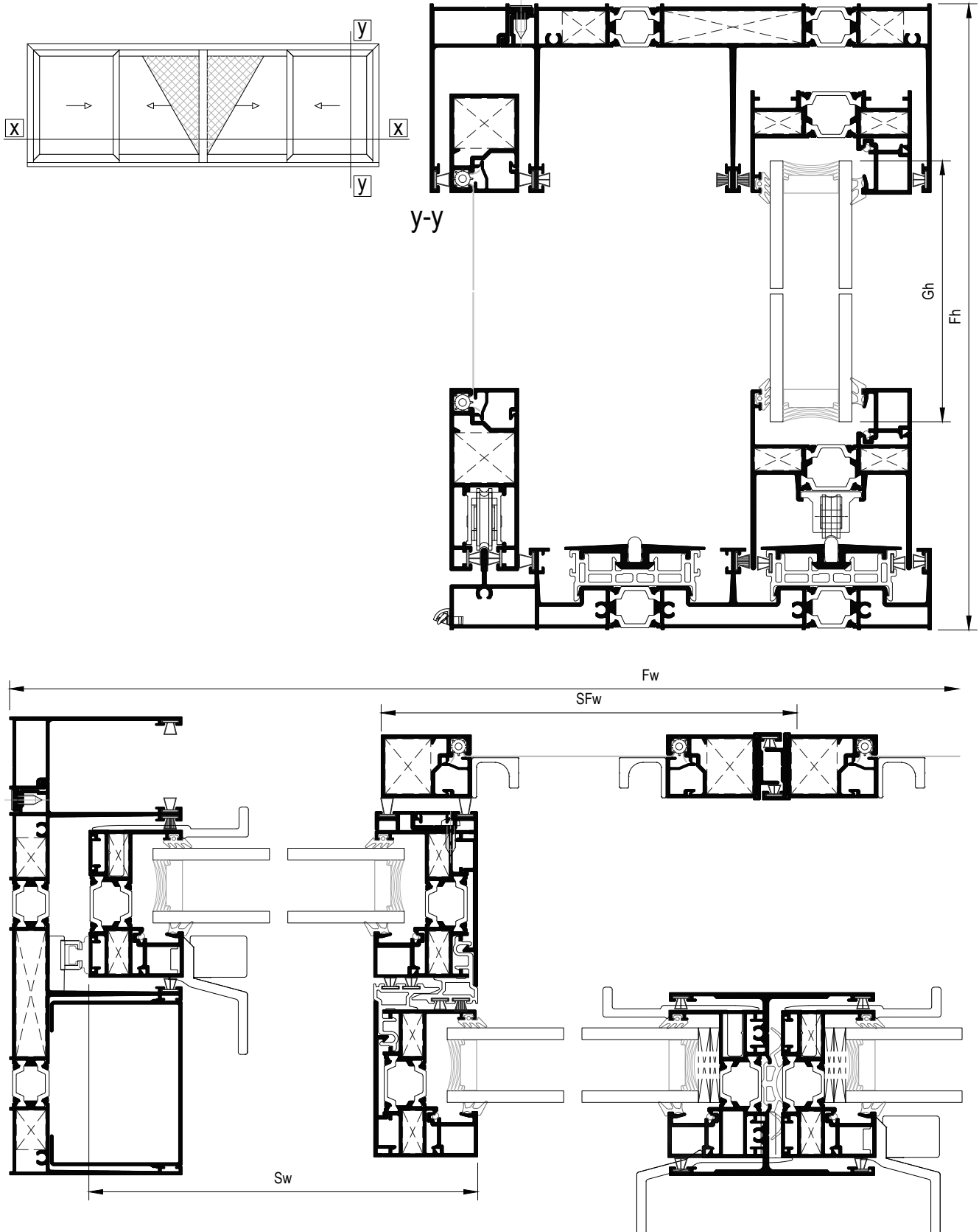
Cf Four-sash meeting stile sliding window with flyscreen Τετράφυλλο φιλητό συρόμενο με σήτα
